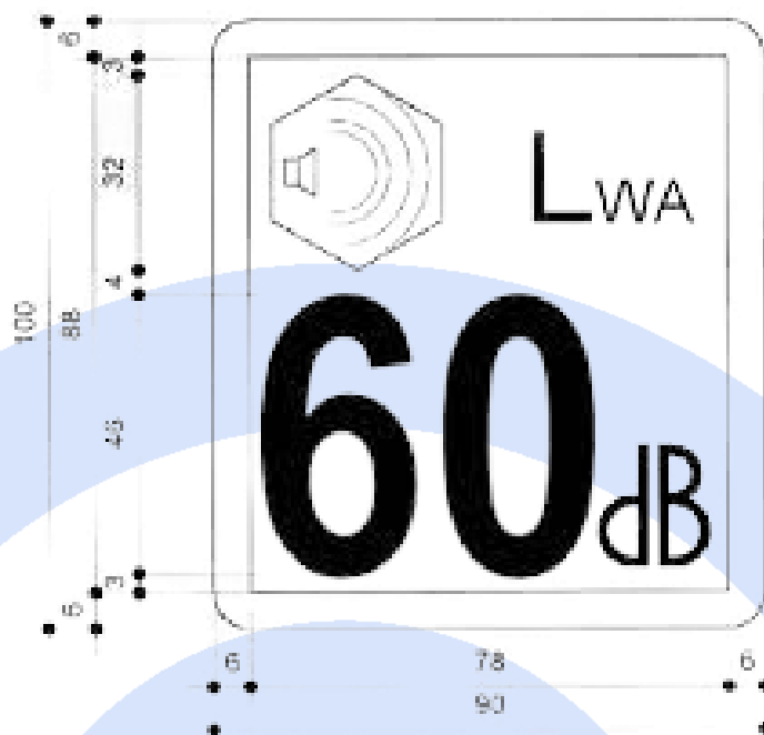
Rysunek 4 Oznaczenie gwarantowanego poziomu mocy akustycznej
